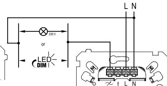
Рис. 3. Подключение к трем проводам
