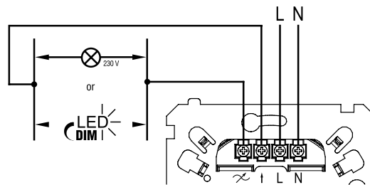
Рис. 2. Подключение к четырем проводам
